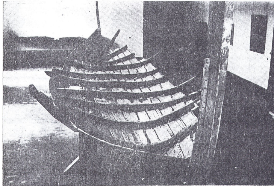
Ryc. 36. Szczątki okrętu z Czarnowska (Charbrów III- wg W. Filipowiaka).
