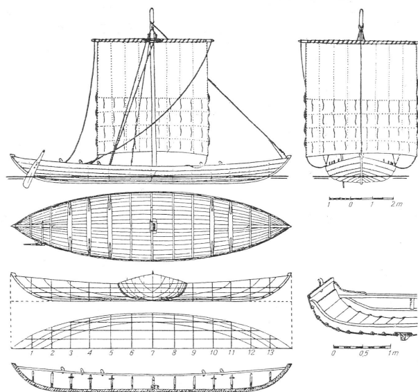
Ryc. 11. Próba rekonstrukcji statku z Charbrowa, na podstawie O. Lienaua, szkice własne.
