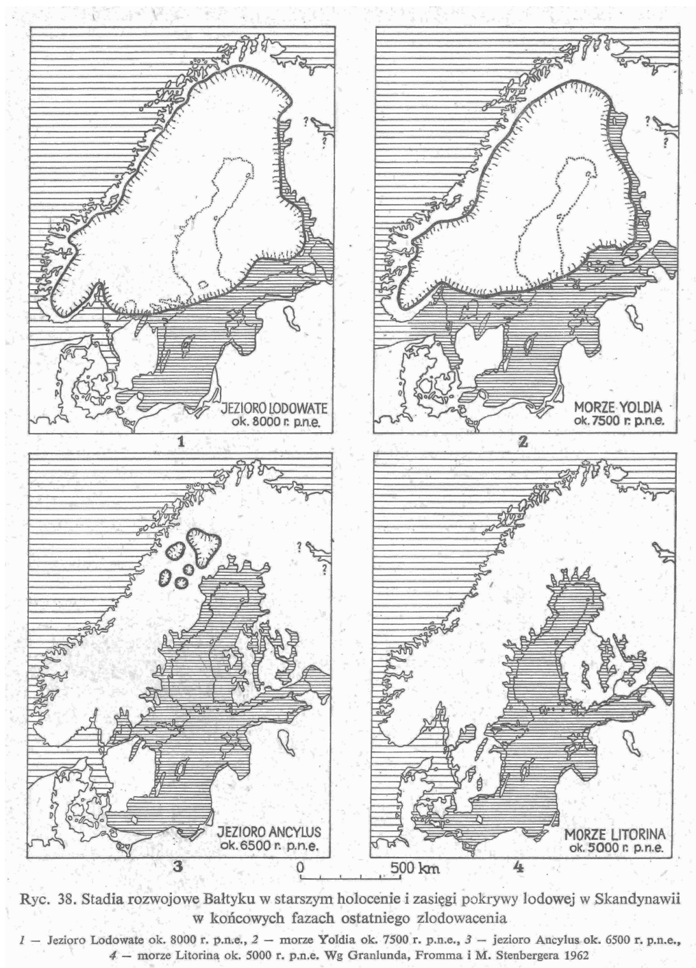
Ryc. 1. Stadia rozwojowe Bałtyku w starszym holocenie i zasięgi pokrywy lodowej w Skandynawii w końcowych fazach ostatniego zlodowacenia 13 .
