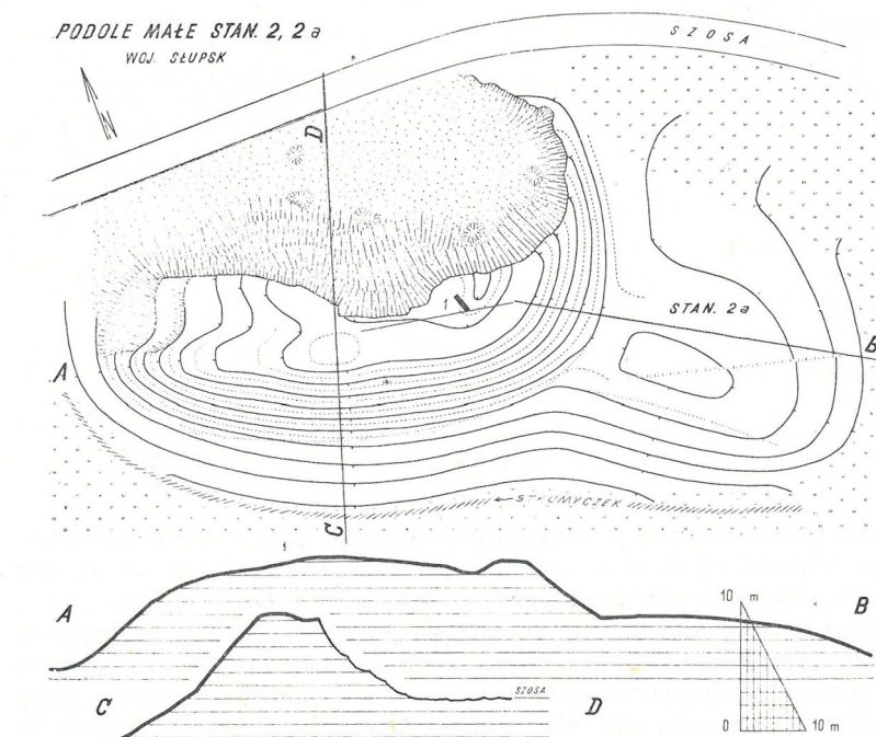
Ryc. 41. Podole Małe, gm. Dębica Kaszubska. Stanowisko 2. Plan warstwicowy grodziska
