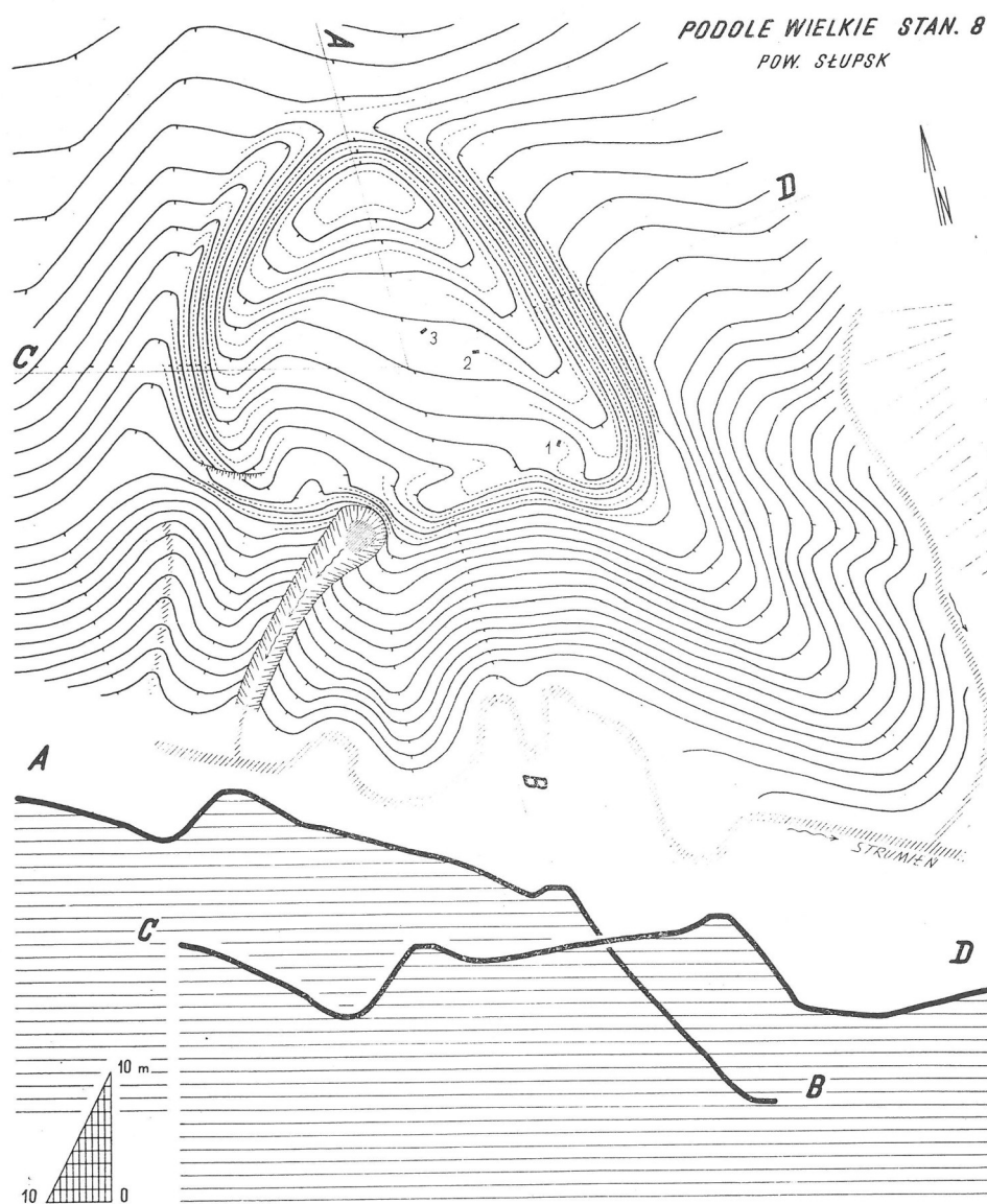
Ryc. 31. Podole Wielkie, pow. Słupsk. Stanowisko 8. Nr kat. 82. Plan warstwiczny grodziska.
