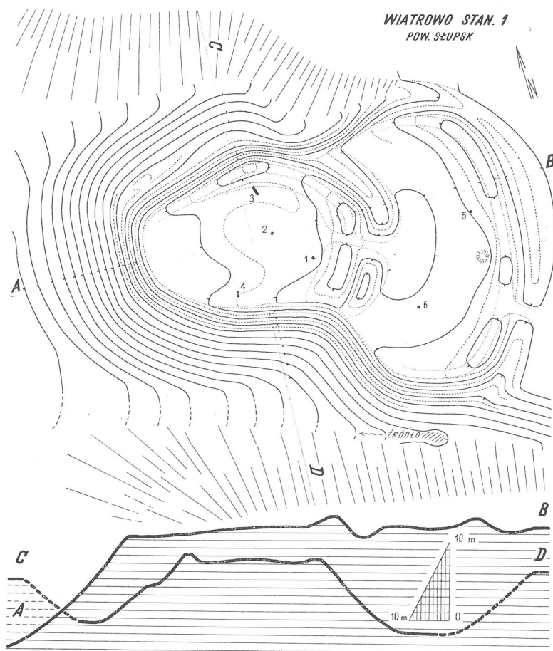
Ryc. 64. Wiatrowo, pow. Słupsk. Stanowisko 1. Nr kat. 143. Plan warstwicowy grodziska.
