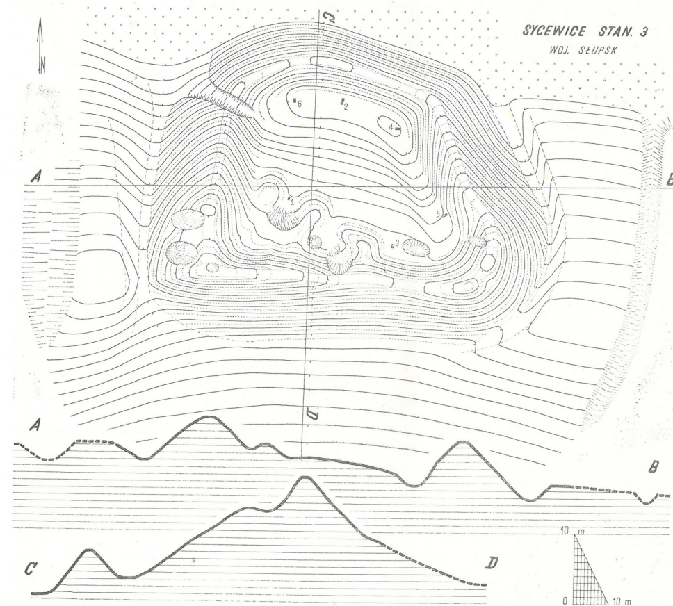
Ryc. 67. Sycewice, gm. Kobylnica, Stanowisko 3. Plan warstwowy grodziska
