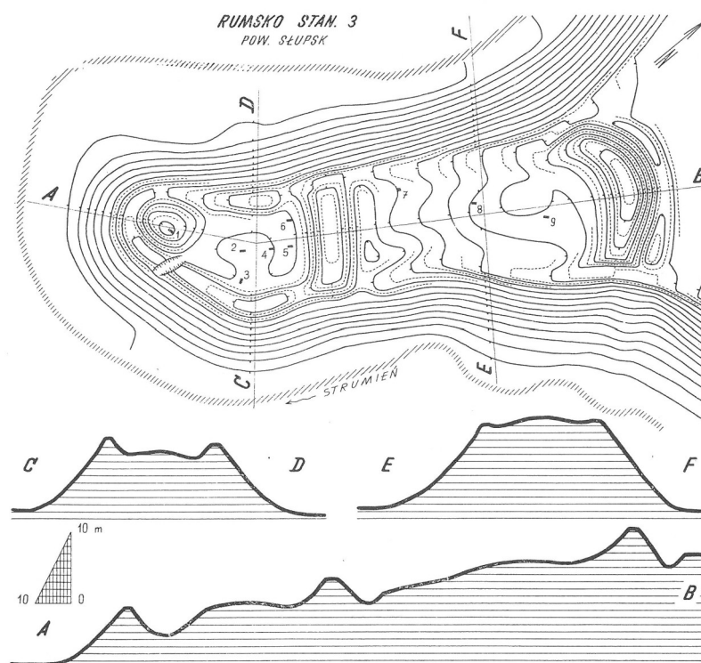
Ryc. 40. Rumsko, pow. Słupsk. Stanowisko 3. Nr kat. 103. Plan warstwicowy grodziska.
