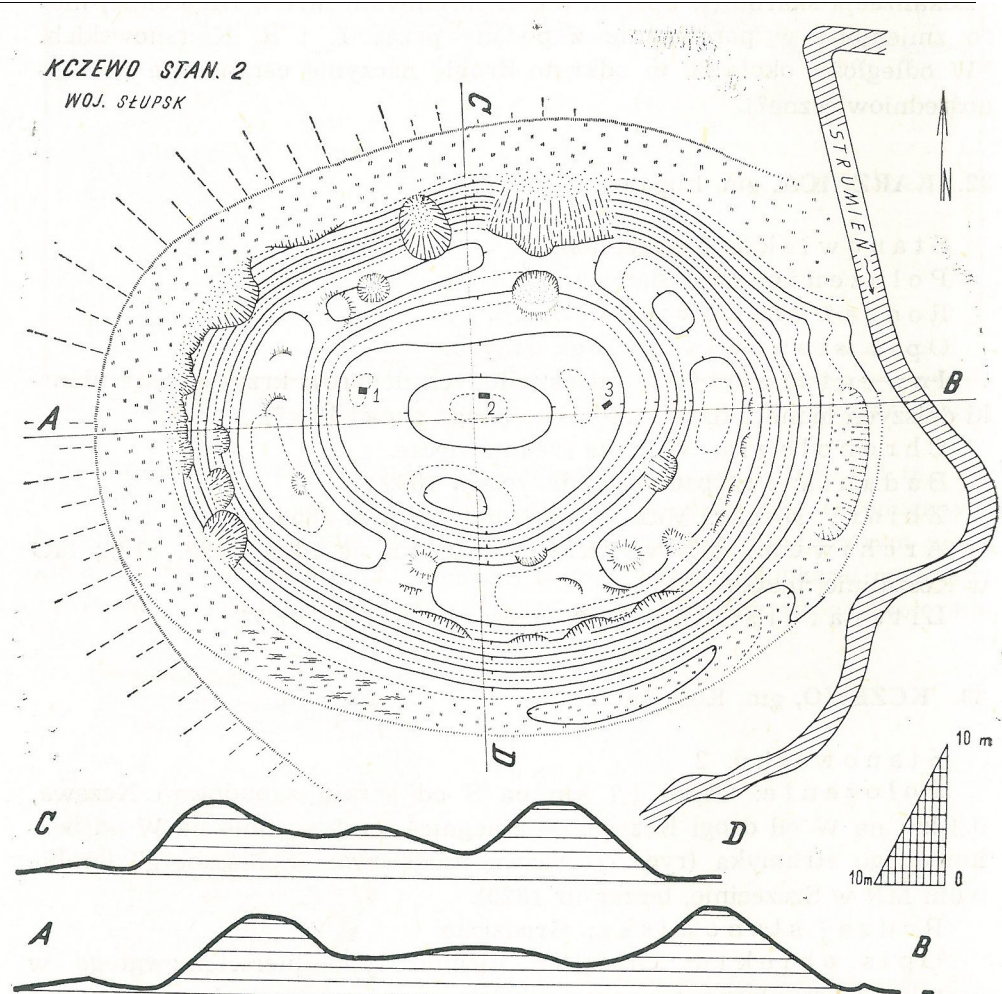
Ryc. 18. Kczewo, gm. Kobylnica, Stanowisko 2. Plan warstwicowy grodziska
