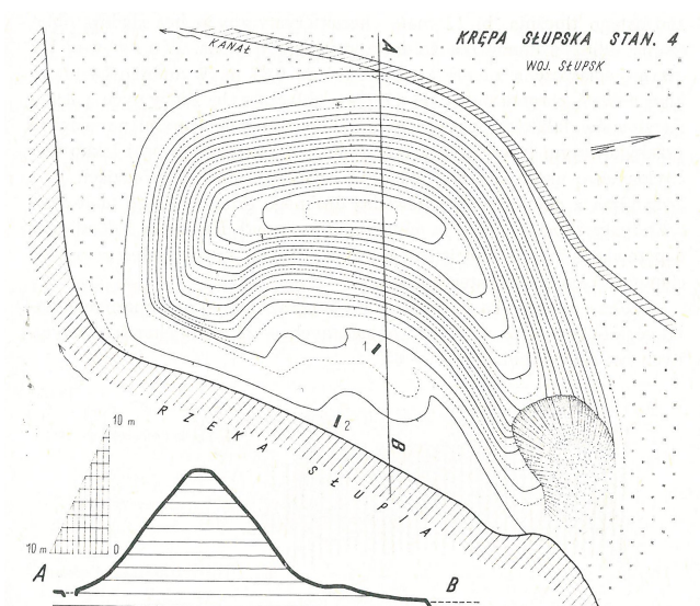
Ryc. 26. Krępa Słupska, gm. Słupsk. Stanowisko 4. Plan warstwicowy grodziska
