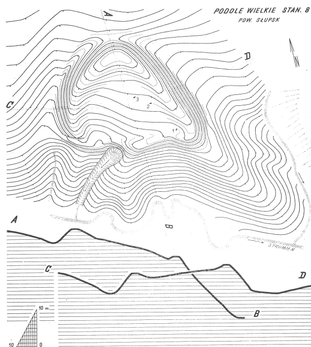
Ryc. 31. Podole Wielkie, pow. Słupsk. Stanowisko 8. Nr kat. 82. Plan warstwicowy grodziska.
