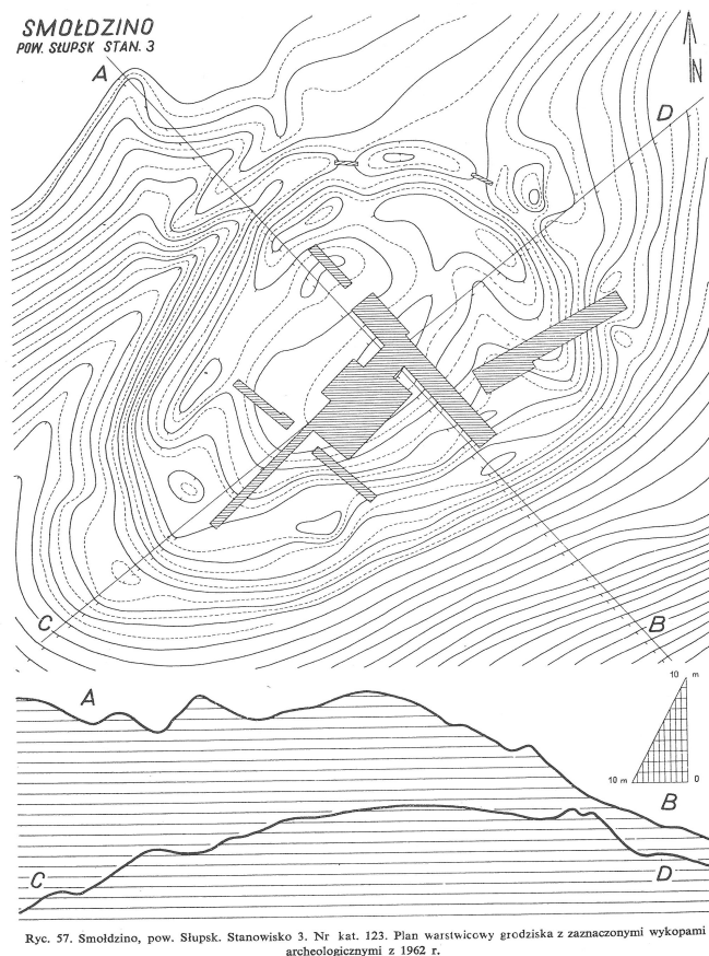
Ryc. 18. Smoldzino. Plan warstwicowy grodziska.
