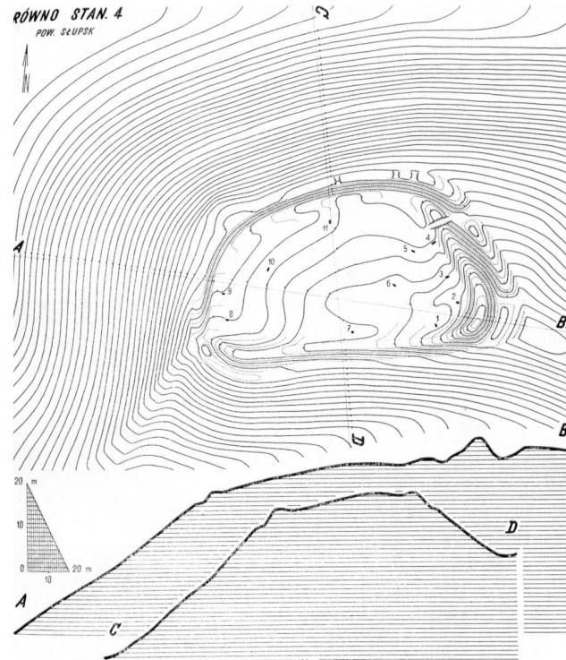
Ryc. 13. Równo. Plan warstwicowy grodziska.
