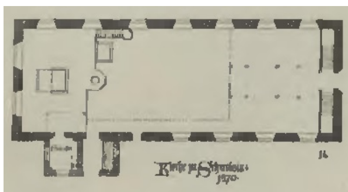
Ryc. 11. Kościół w Smoldzinie- rzut przyziemia. Stan 1870 r. Źródło: Ludwig Böttger, Die Bau- u. Kunstdenkmäler der Provinz Pommern. T. 3, Bd.2, H. 4, Kreis Stolp. Stettin 1894, s. 27.
